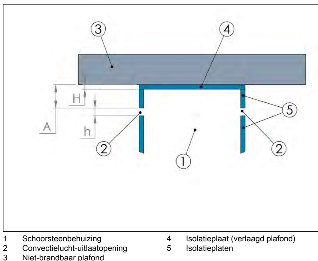
Figuur 14. Afstanden tot niet-brandbaar plafond – Vooraanzicht
