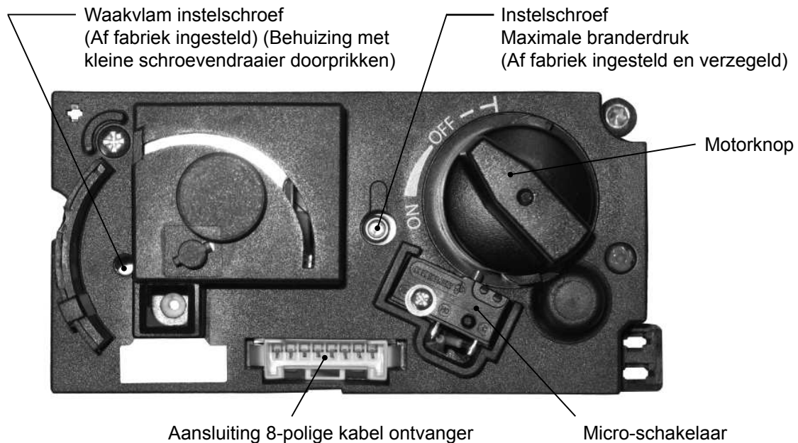
Figuur 4: Gasregelblok
