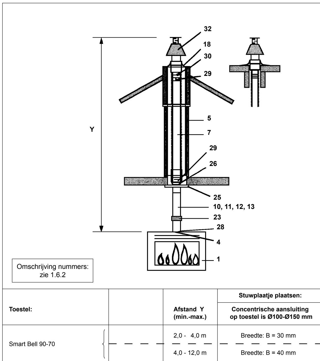
Figuur 6: Verticale schoorsteenuitmonding bij gebruik van een bestaand rookkanaal (Flexibel Ø100 mm en/of star Ø100 mm / Ø 150 mm)
