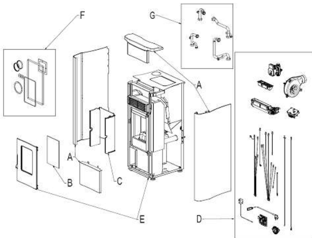
Fig. 1 - Geëxploodeerde tekening
