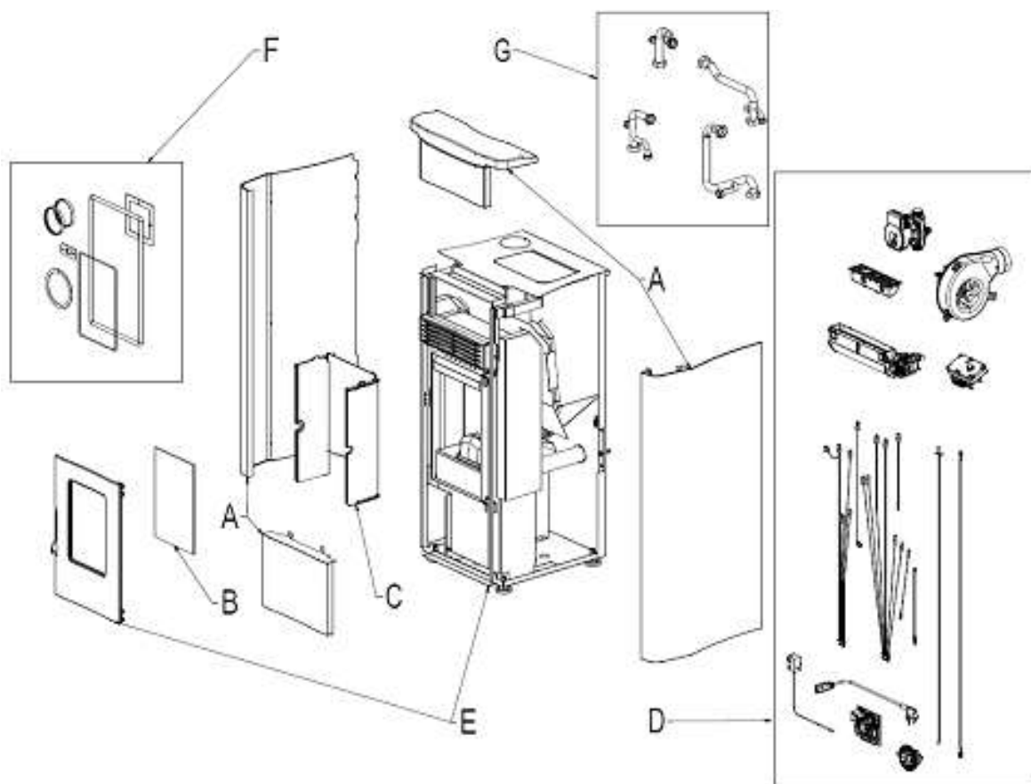
Fig. 1 - Geëxplodeerde tekening
