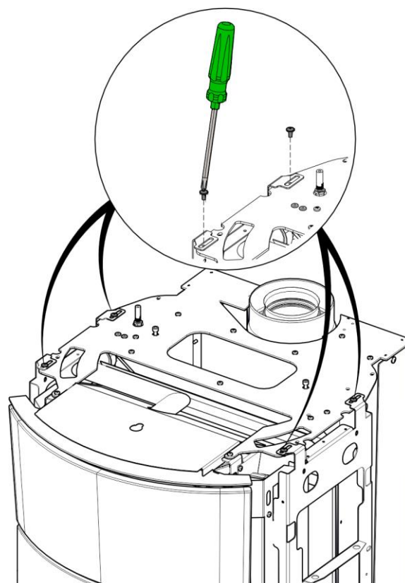
3) Draai de schroeven los
