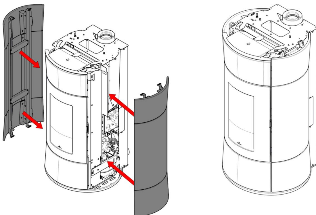
Geassembleerd zijpaneel
