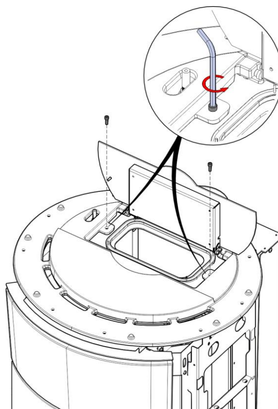
1) Open het pelleteservoir en draai de schroeven los
