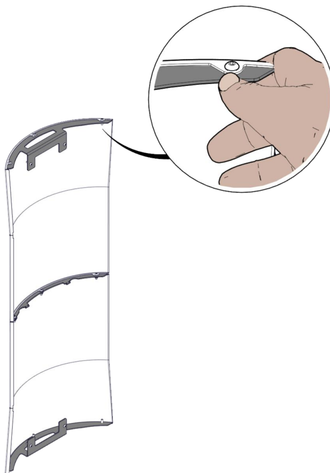
Detail van de plaatsing van de beugels
