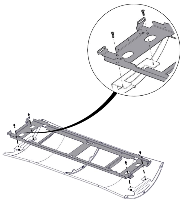
5) Plaats metalen steun
