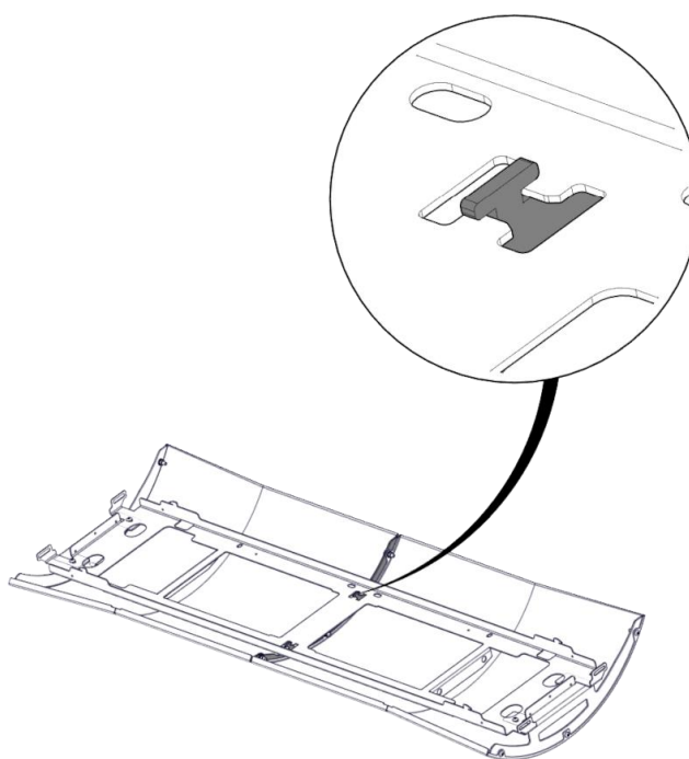
Detail van inzetten van metalen steun
