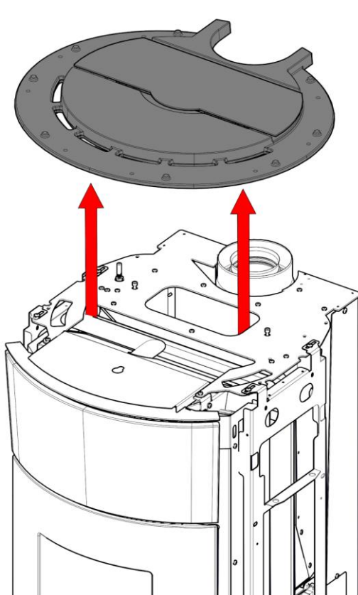
2) Til de bovenkant op
