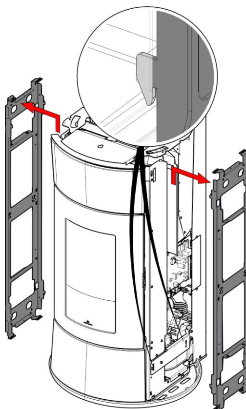
4) Gedemonteerde zijwand
