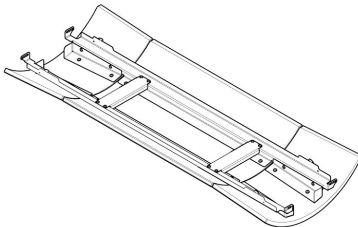
Geassembleerd zijpaneel
