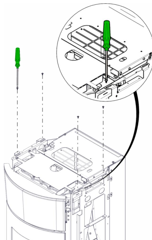
3) Draai de schroeven los
