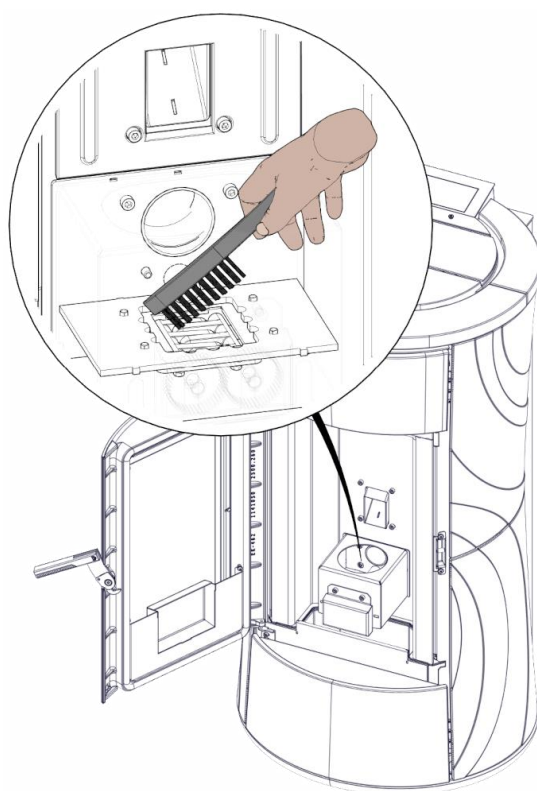
5) Reinig de “KAMMEN” zorgvuldig om te voorkomen dat vervuiling het systeem blokkeert.
