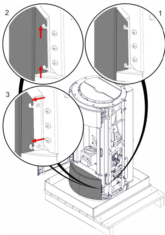
2) Verwijdering voorpaneel
