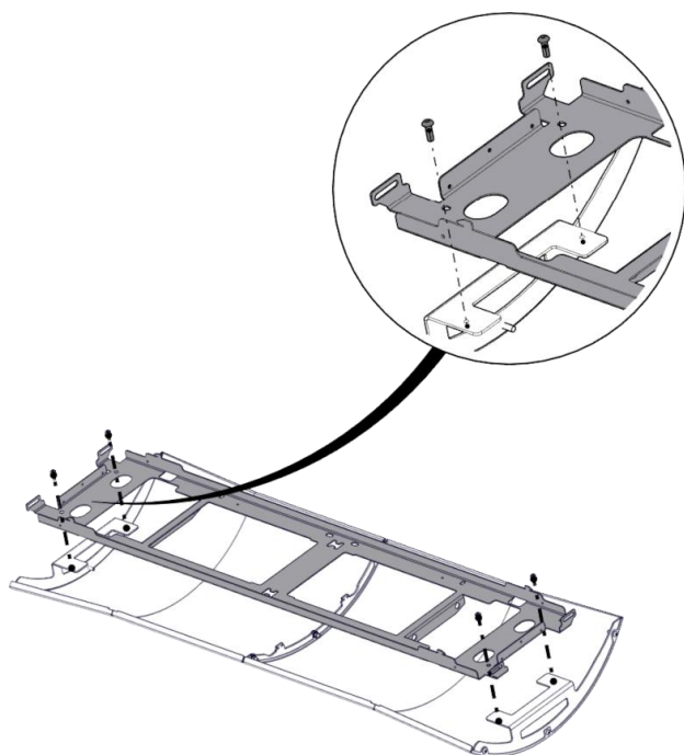
5) Plaats metalen steun
