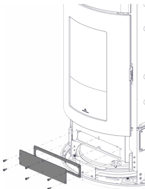
6) Schroef de schroeven los en verwijder het metalen voorpaneel
