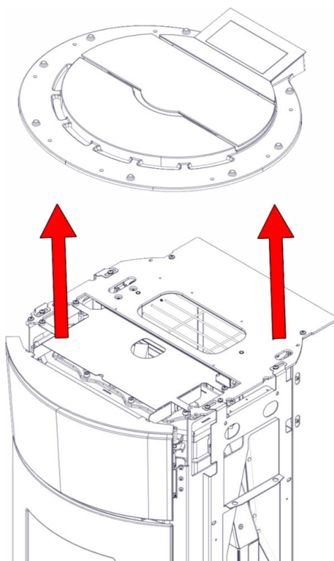
2) Til de bovenkant op
