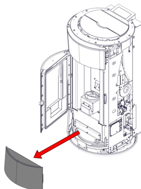
5) Voorpaneel verwijderd
