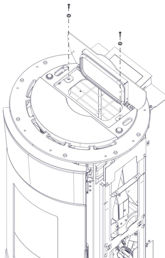
1) Open het pelletreservoir en draai de schroeven los
