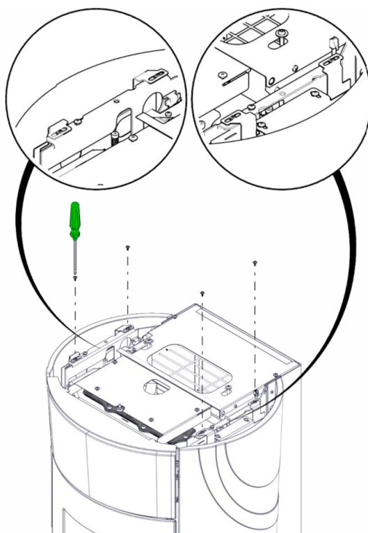
3) Haal de zijpanelen eraf
