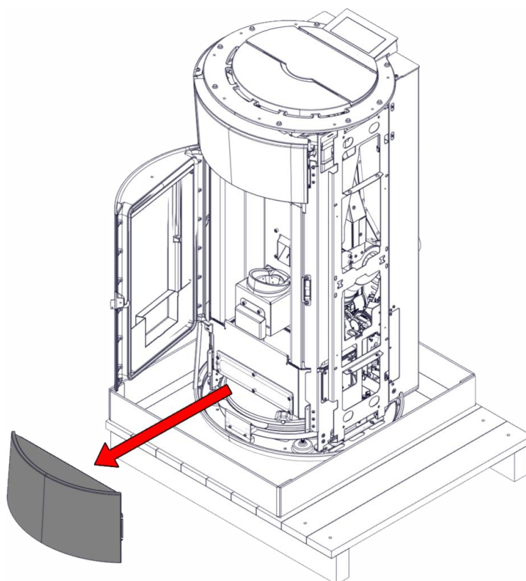
Voorpaneel verwijderd
