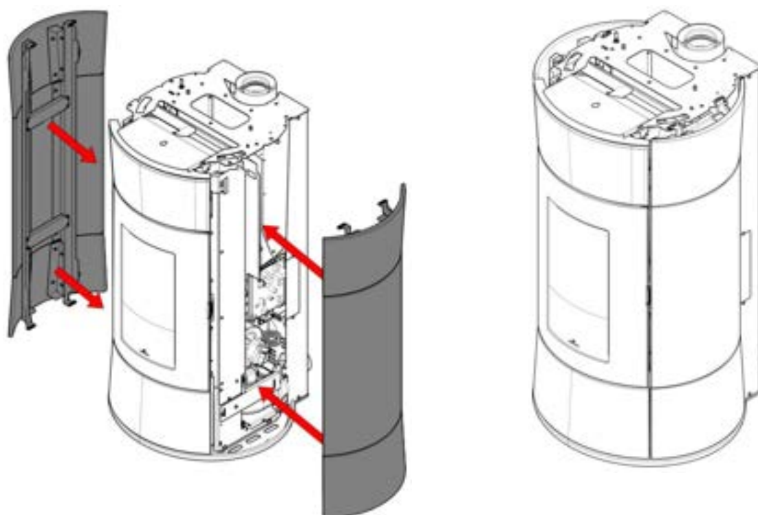
Geassembleerd zijpaneel
