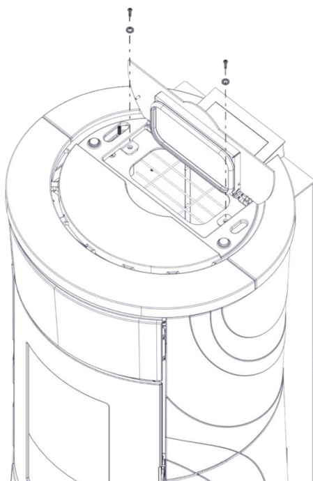
1) Open het reservoir en draai de schroeven los
