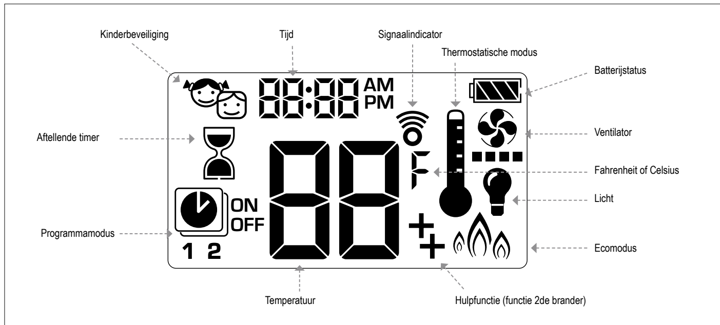
Afbeelding 2: 10-symbolendisplay
