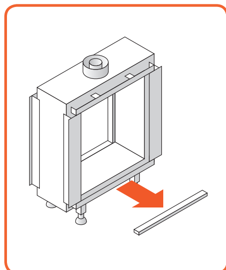
Afbeelding 10.5 - Verwijderen onderlijst
