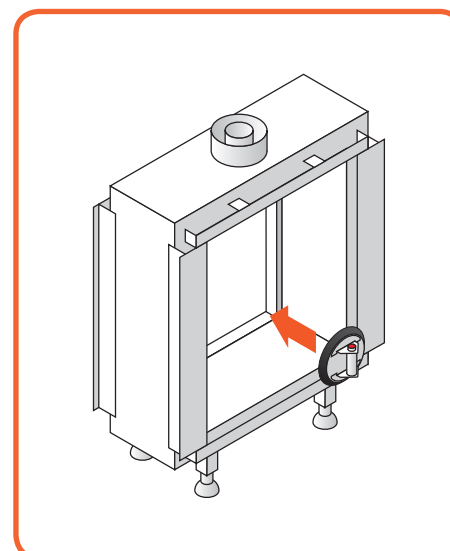
Afbeelding 10.8 - Opzetten zuignap
