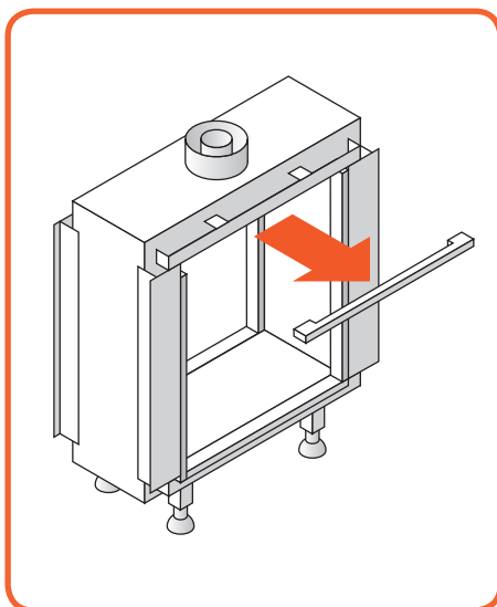
Afbeelding 10.3 - Verwijderen bovenlijst
