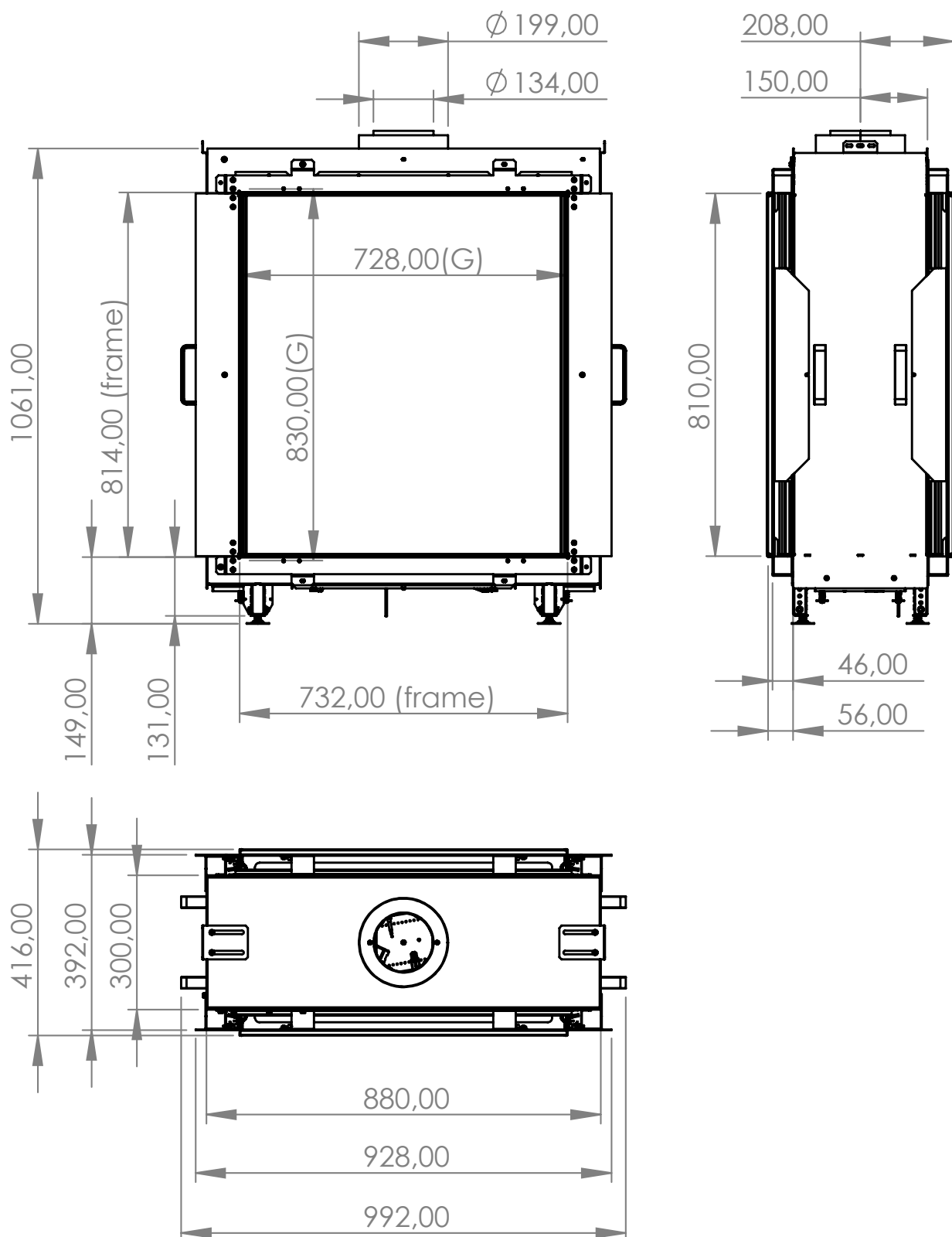
Afbeelding 1.2 - Lijntekening Sky Small T
