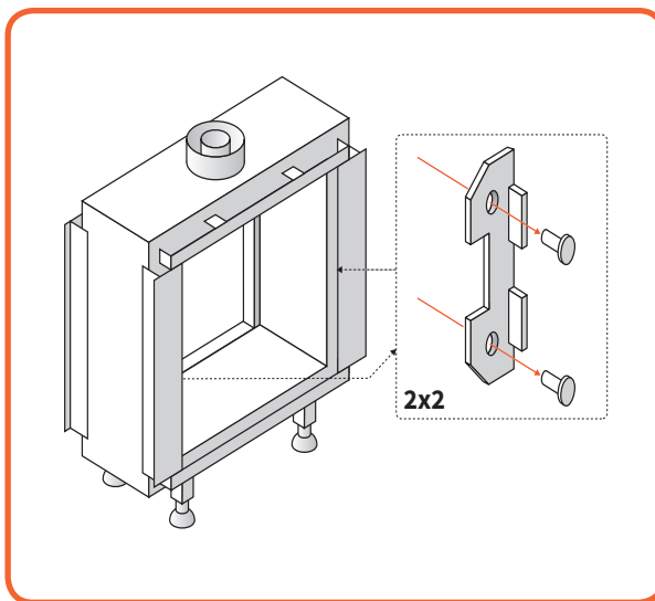
Afbeelding 10.6 - Verwijderen klemmen
