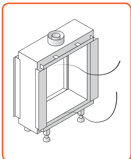
Afbeelding 10.7 - Uithalen glaskoorden
