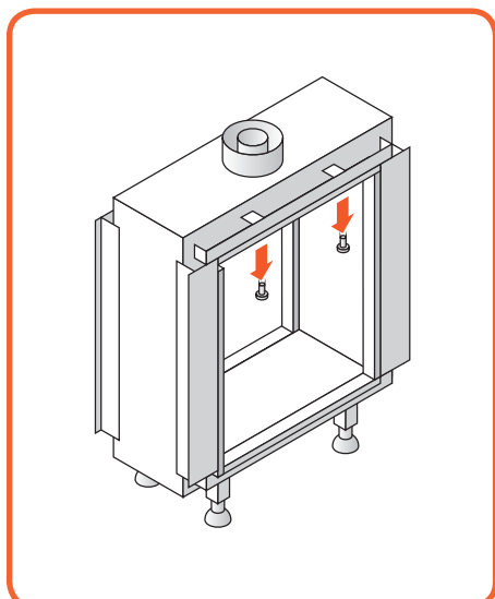
Afbeelding 10.2 - Verwijderen schroeven
