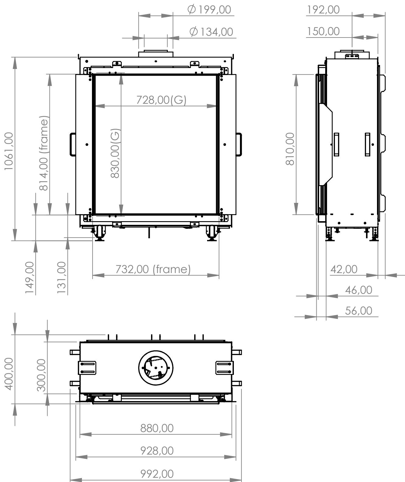
Afbeelding I.1 - Lijntekening Sky Small F
