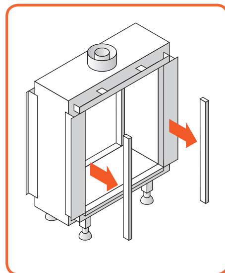
Afbeelding 10.4 - Verwijderen zijlijsten
