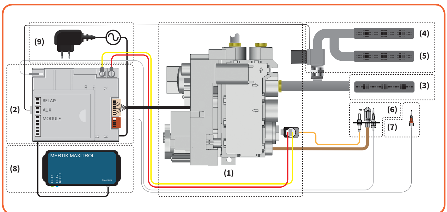
Afbeelding 9.1 - Electronisch schema van de Sky Small
