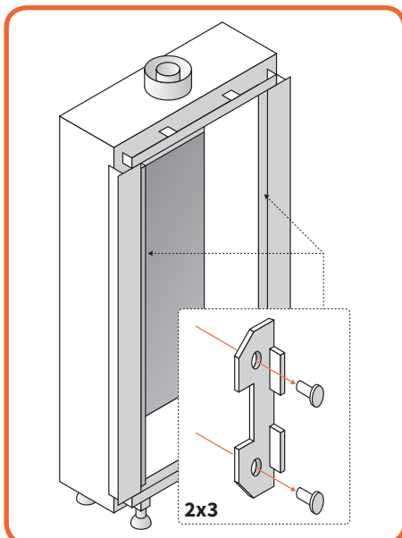
Afbeelding 10.6 - Verwijderen klemmen
