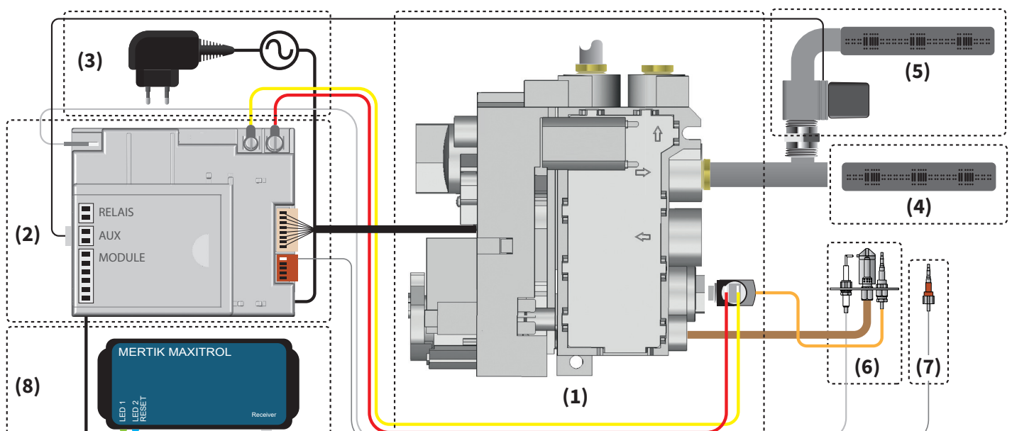
Afbeelding 9.1 - Electronisch schema van de Sky(-T)
