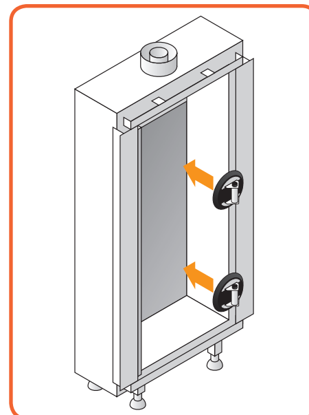
Afbeelding 10.8 - Opzetten zuignap
