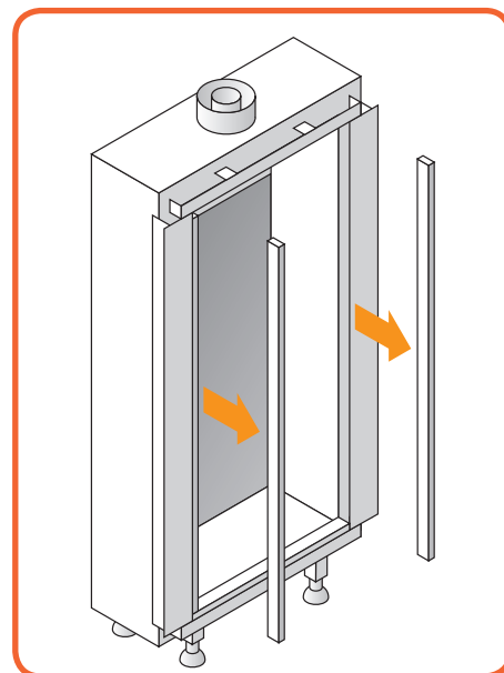
Afbeelding 10.4 - Verwijderen zijlijsten
