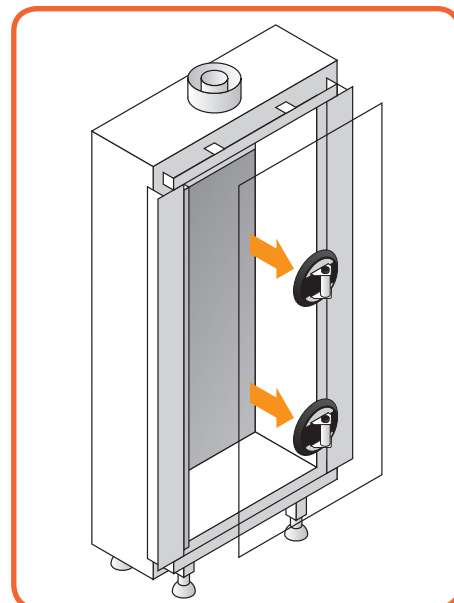
Afbeelding 10.9 - Uithalen glas
