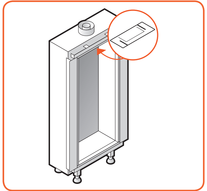
Afbeelding E.1 - Positie Rookgasbegrenzer Sky (-T)
