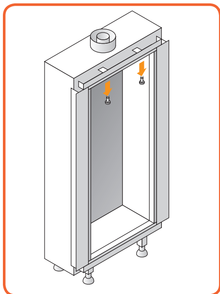
Afbeelding 10.2 - Verwijderen schroeven
