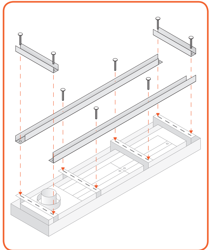
Afbeelding 6.10 - Creëer een frame op de profielen van de haard
