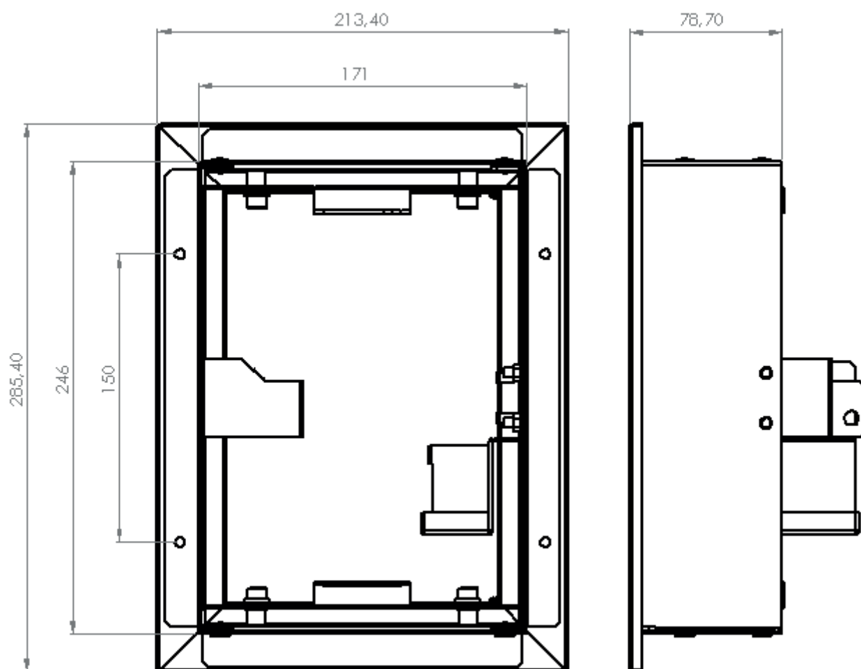
Afbeelding I.1 - Bedieningsluik, BDLE4
