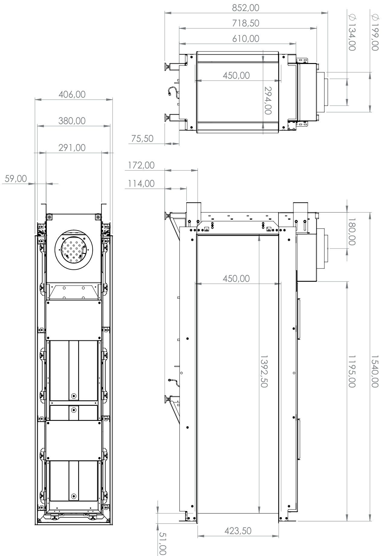
Afbeelding I.5 - Lijntekening Summum 140 RD
