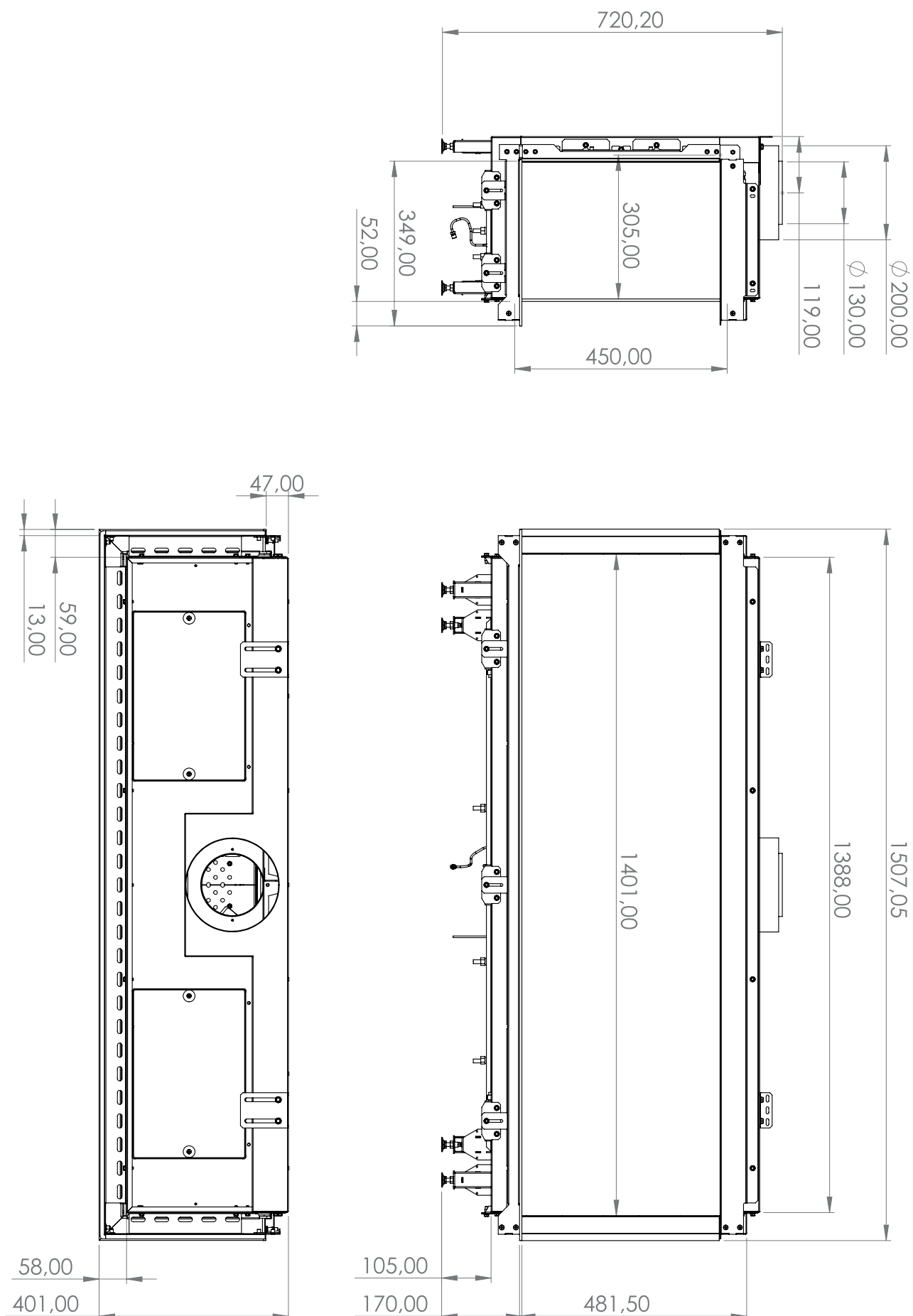
Afbeelding I.4 - Lijntekening Summum 140 3S
