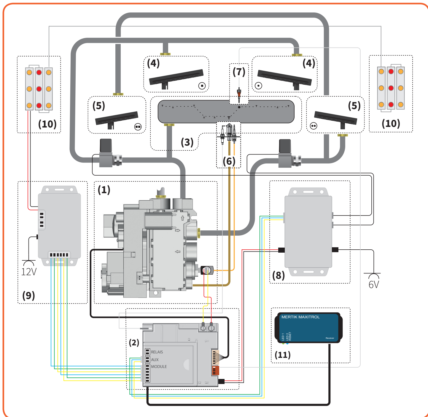
Afbeelding 9.1 - Electronisch schema van de Summum 140 modellen
