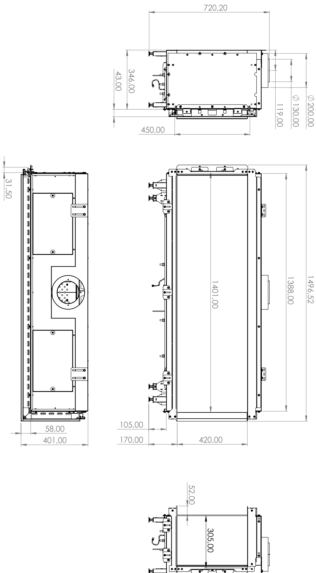
Afbeelding I.3 - Lijntekening Summum 140 C
