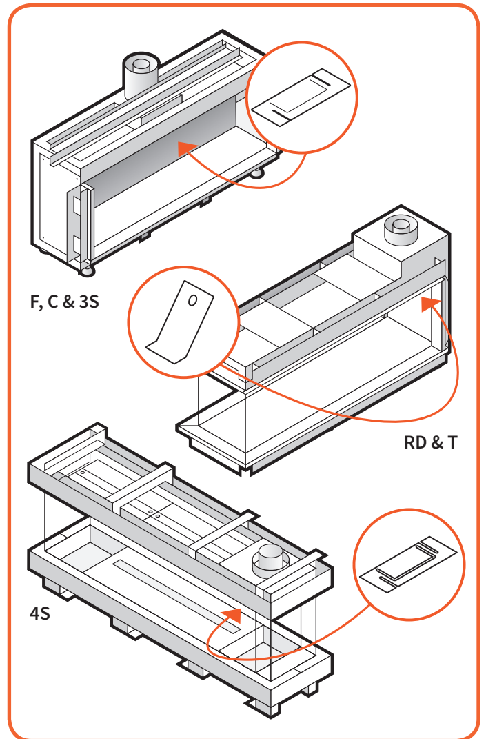
Afbeelding E.1 - Positie Rookgasbegrenzer Summum 140
