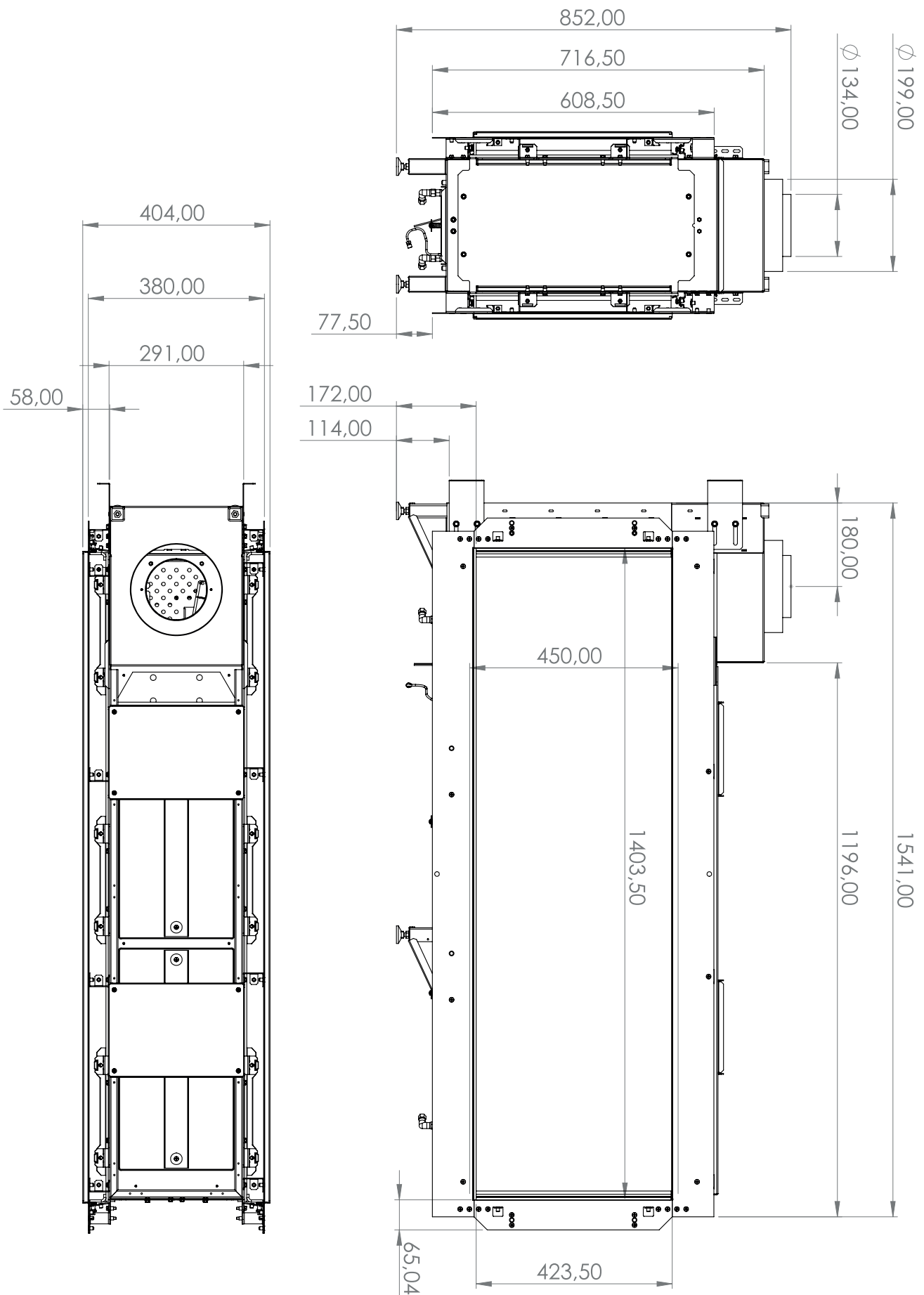
Afbeelding 1.6 - Lijntekening Summum 140 T
