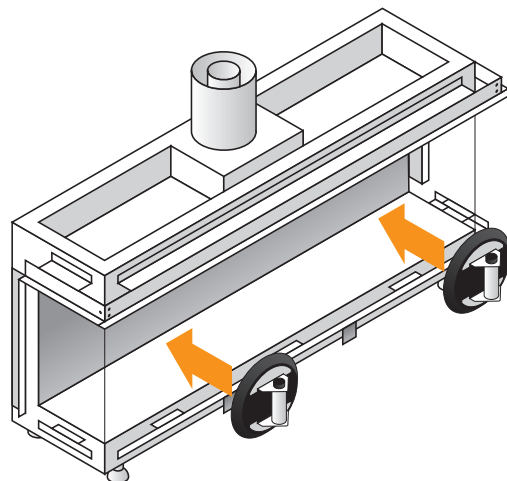
Afbeelding 10.5 - Opzetten van de zuignap
