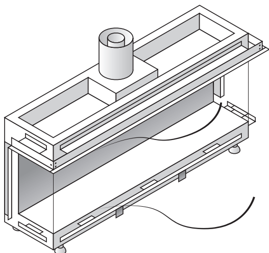
Afbeelding 10.4 - Verwijderen van de glaskoorden
