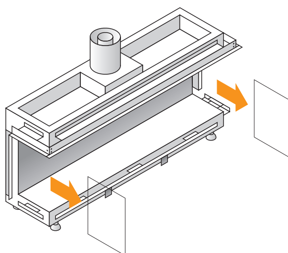
Afbeelding 10.7 - Verwijderen van de zijruiten waar nodig
