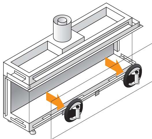
Afbeelding 10.6 - Uithalen van het glas
