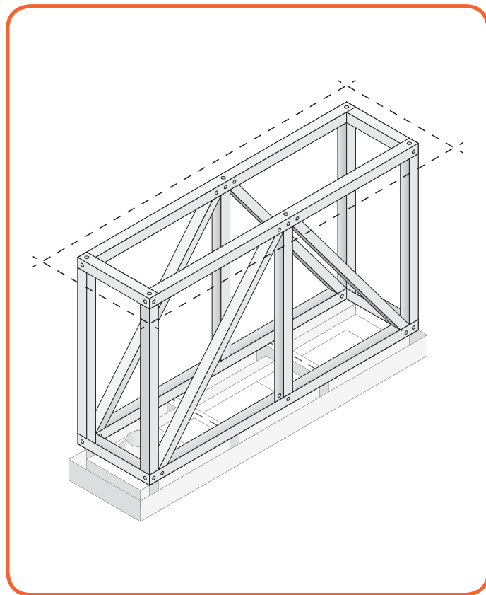
Afbeelding 6.15 - Eindresultaat ophanging
