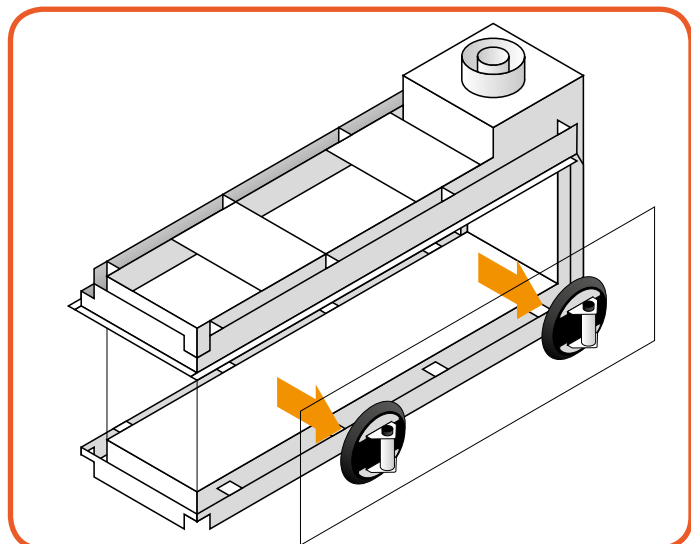
Afbeelding 10-6: Uithalen van het glas
