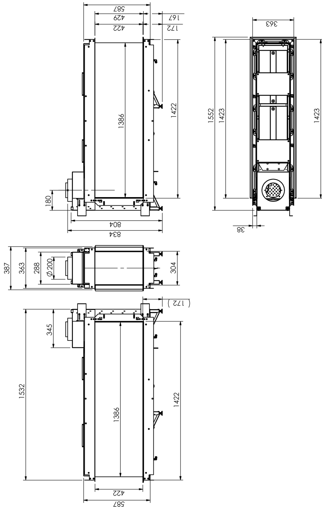
Afbeelding I-2: Lijntekening Lucius 140
