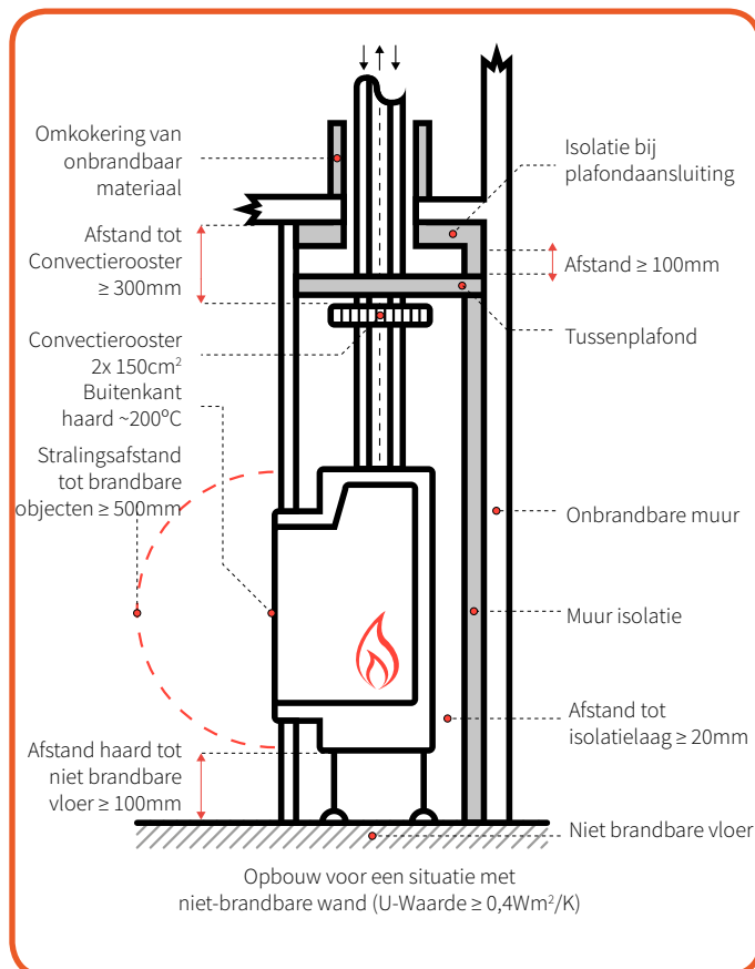
Afb. 6-1: Niet-brandbare wand-/dakmateriaal
