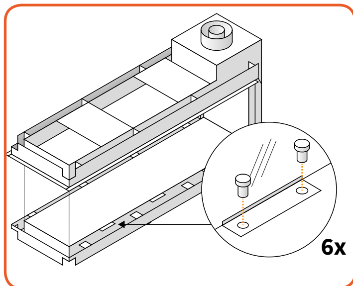
Afbeelding 10-4: Verwijderen schroeven van de glasklemmen
