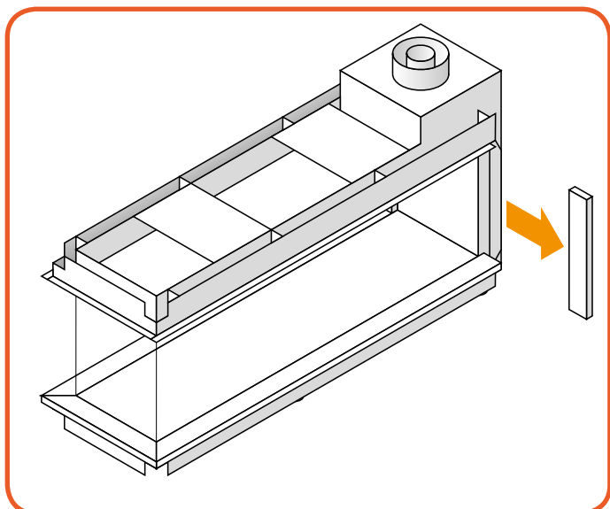
Afbeelding 10-2: Verwijderen zijlijsten Lucius*
