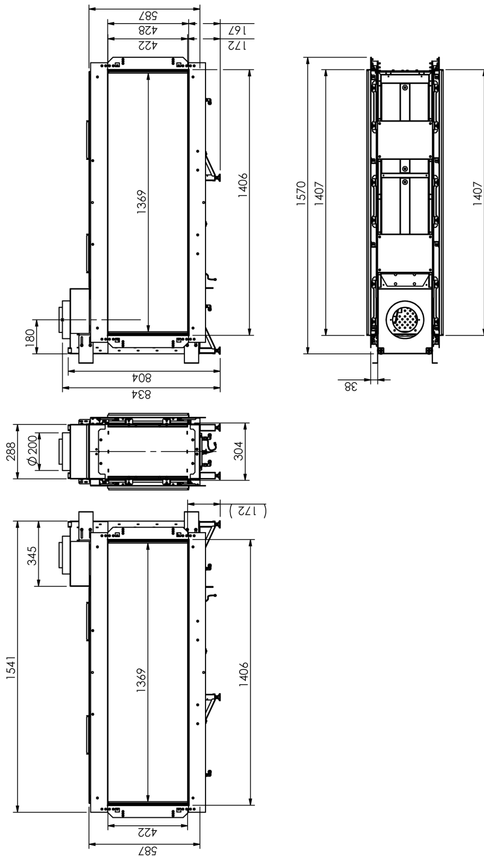
Afbeelding I-3: Lijntekening Tenore140
