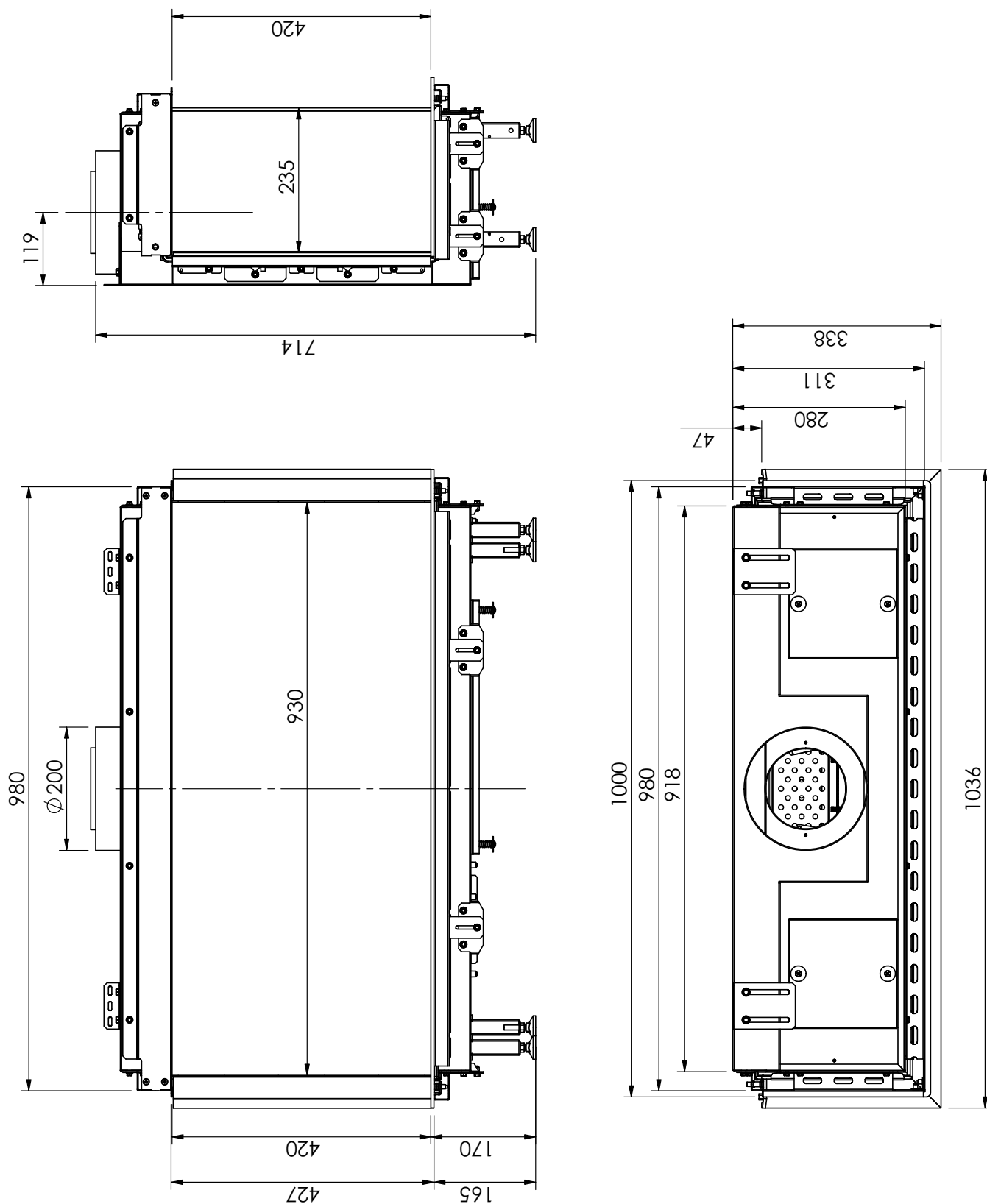
Afbeelding I-4: Lijntekening Trisore100
