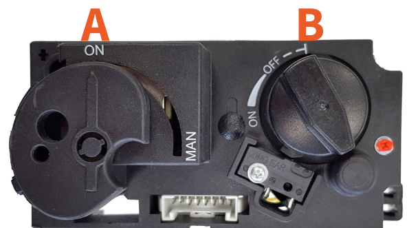
Afbeelding 4-3: Hoofdbrander ontsteking
