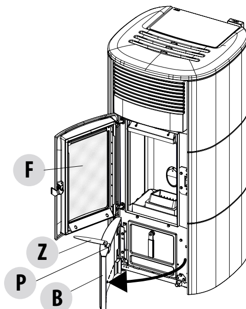
ONDERSTE DEUR OPENEN
