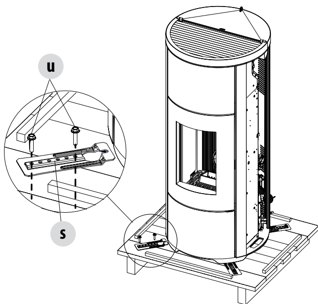
VERWIJDERING BEVESTIGINGSBEUGELS
