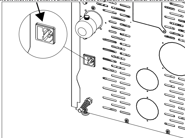
ELEKTRISCHE AANSLUITING VAN DE KACHEL
