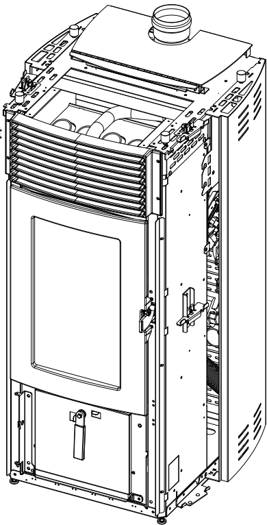
KACHEL STAR ZONDER BEKLEDING
