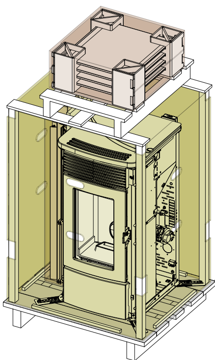
VERPAKKING ALYSSA MET BEKLEDING IN KERAMIEK
