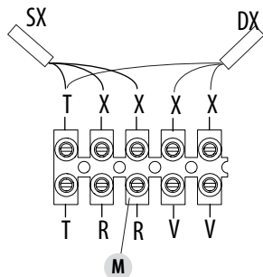
Figuur 8 – Positie kabels op het klemmenbord
