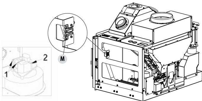
Figuur 7 – Positie klemmen ventilatoren
