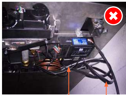
led-modulekabel ontsteekkabel
