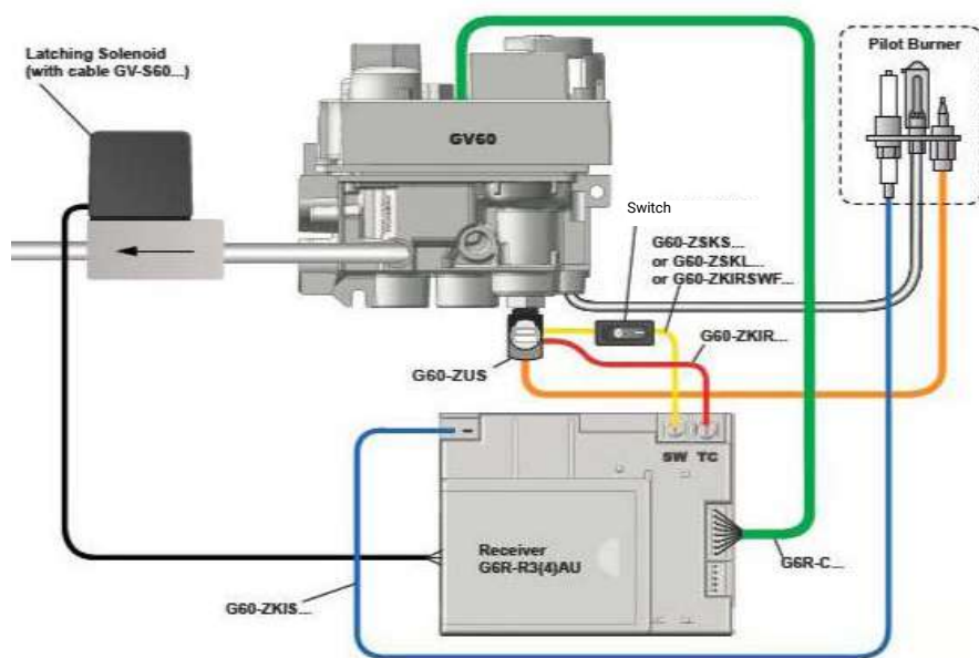
Schematische voorstelling.
